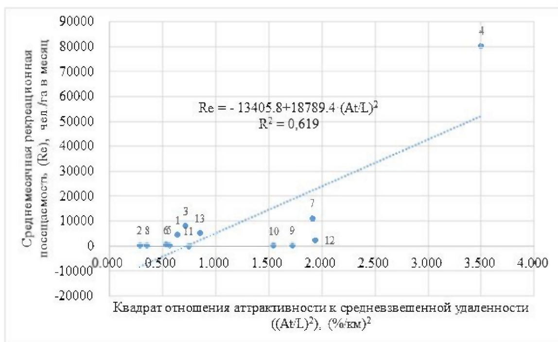
Рис. 1. Регрессионная зависимость рекреационной посещаемости СНП от аттрактивности и удаленности (1 - «33 водопада», 2 - Водопады «Шапсуг-Псыдах», 3 - «Корыта», 4 - Смотровая башня на горе Ахун, 5 - Волконское ущелье, 6 - «Берендеево царство», 7 - Агурское ущелье и водопады, 8 - Водопад «Чудо-Красотка», 9 - Змейковское ущелье и водопады, 10 - Маршрут «Ажек», 11 - Комплекс «Воронцовский», 12 - Белые скалы, 13 - Византийский храм).
