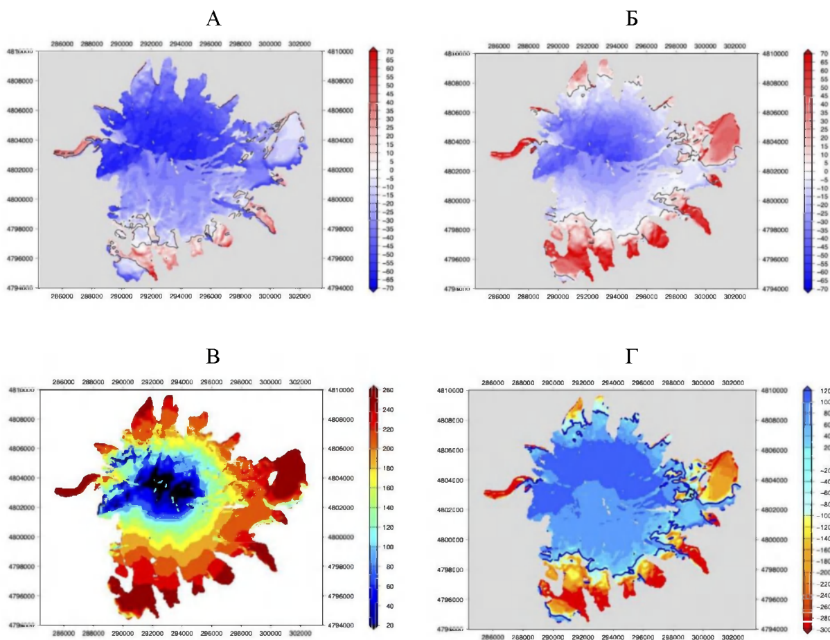
Рисунок 3 – Результаты расчетов согласно сценарию RCP2.6 для десятилетия 2051–2060 гг.: А, Б – радиационный баланс на поверхности ледника, Вт m^{-2} , в среднем за год (А) и июль (Б), тонкой сплошной линией показано положение нулевого баланса; В – количество дней с абляцией; Г – поверхностный баланс массы, мм водн. экв., сплошной синей линией показана снеговая линия, черной – снеговая линия в контрольном эксперименте.
